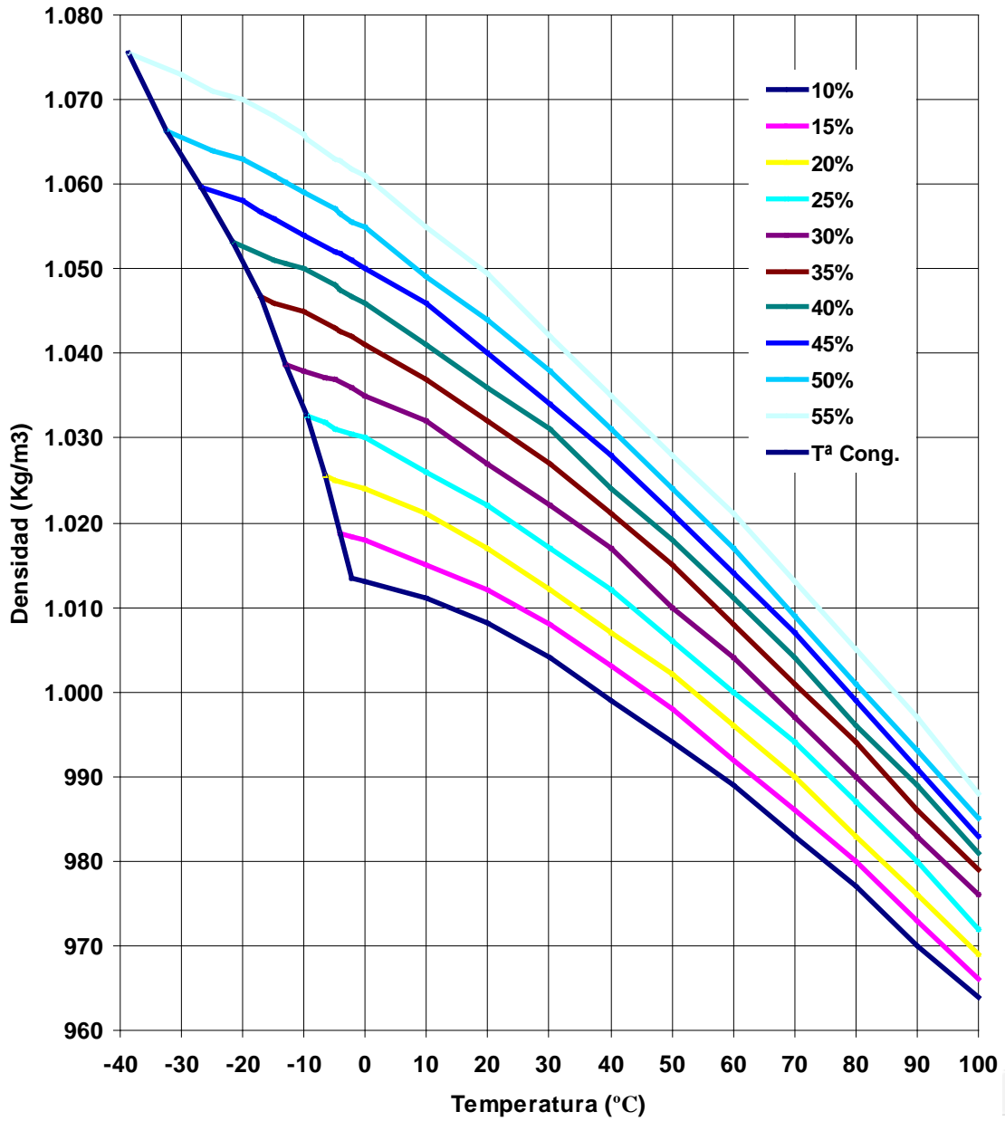
Densidad .vs. % Blue Sun y Tª
