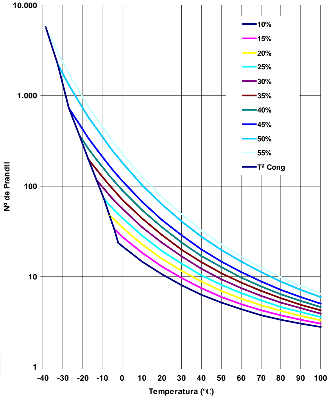
Nº de Prandtl .vs. Blue Sun y T a
